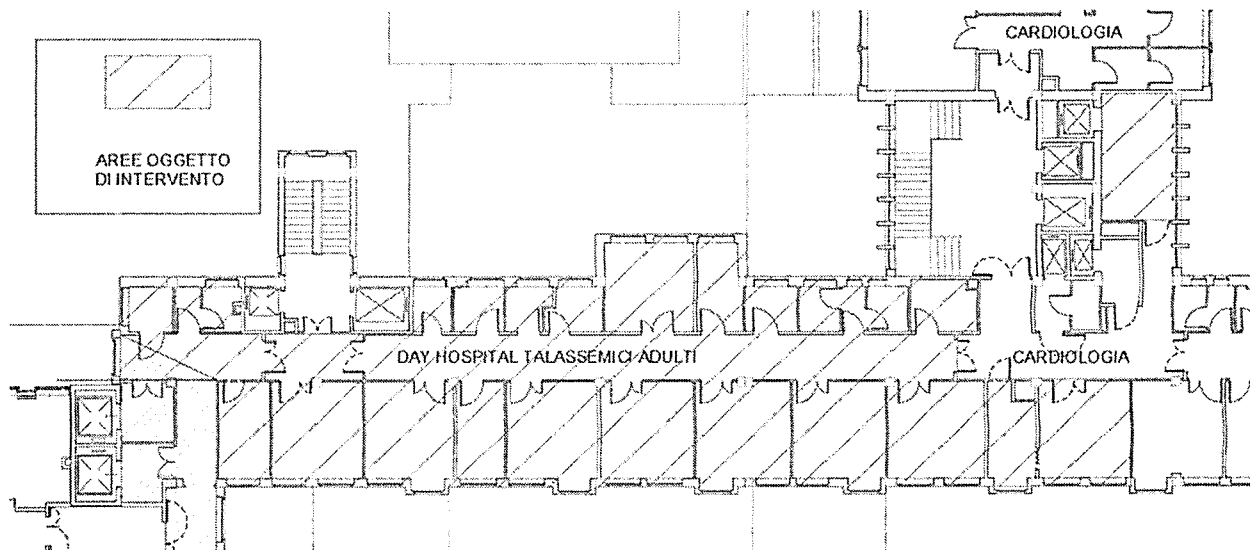
Fig. 1 - Terzo Piano Corpo centrale, ala vecchia P.O. Microcitemico - Aree oggetto di intervento
